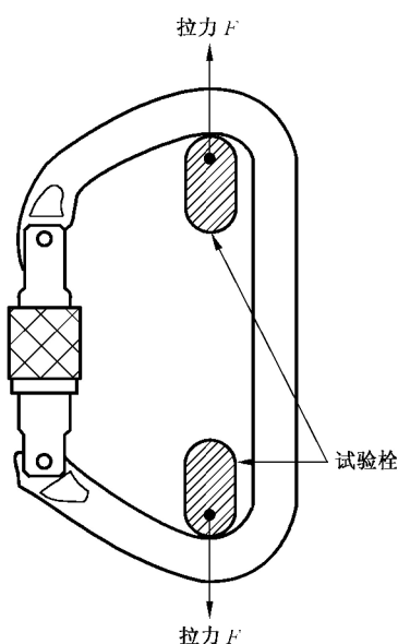
图 2 安全钩开口闭合状态长轴方向破断强度测试示例
