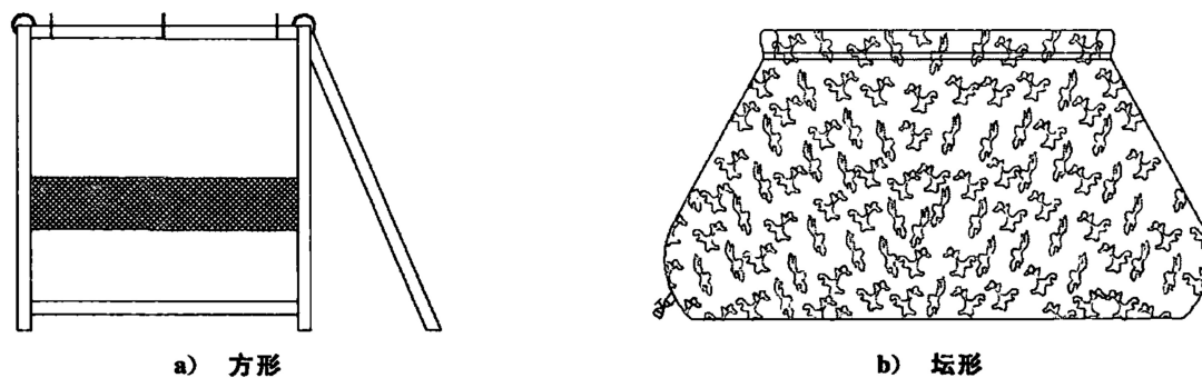
图 A.2 非囊式消防储水装置储水后结构型式
